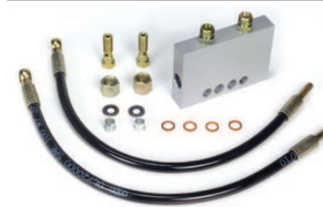
Vandalizm önleyici valf (*) Kol zorlanırsa hidrolik sistemi korur
